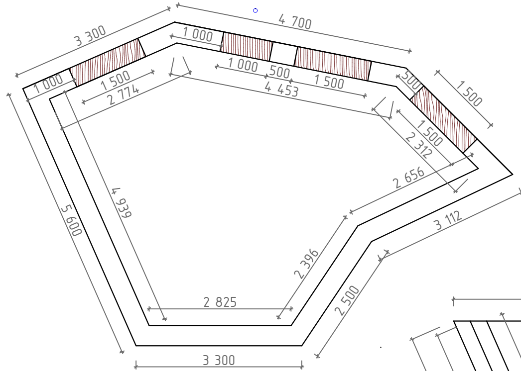
Бетонный борт цветника с местами для сидения
