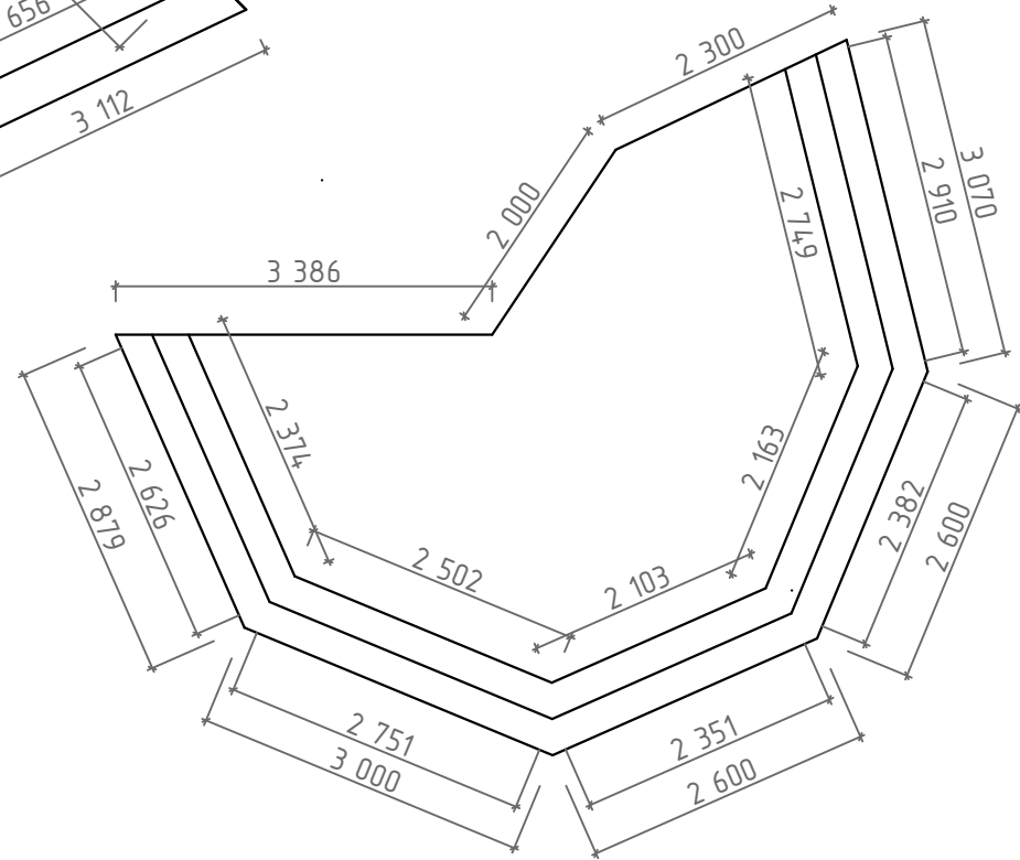
Сцена со ступенями
