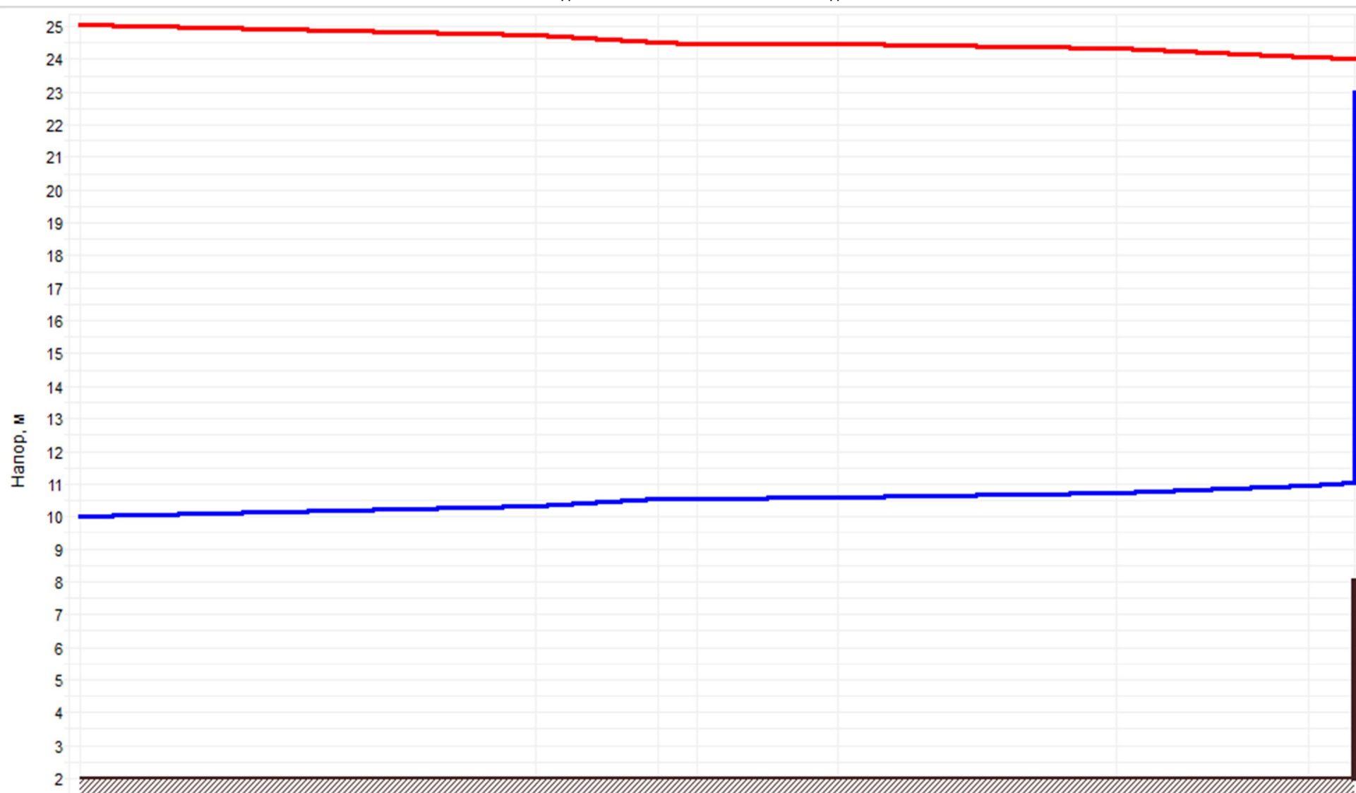
Рисунок 30.2 –График гидравлических режимов рассматриваемого теплопровода
