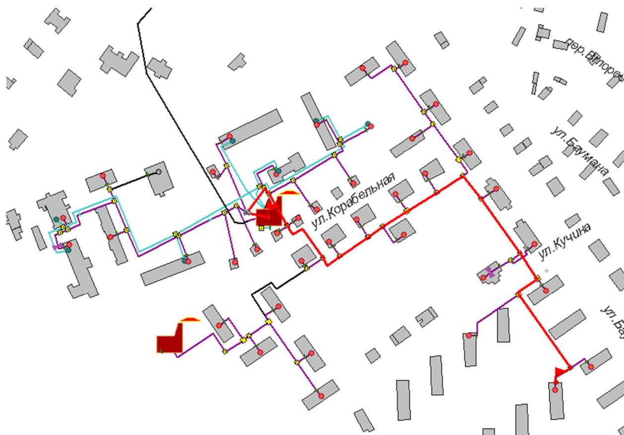
Рисунок 29.1 -Расчетный путь теплоносителя котельной до Баумана,12 к.4
