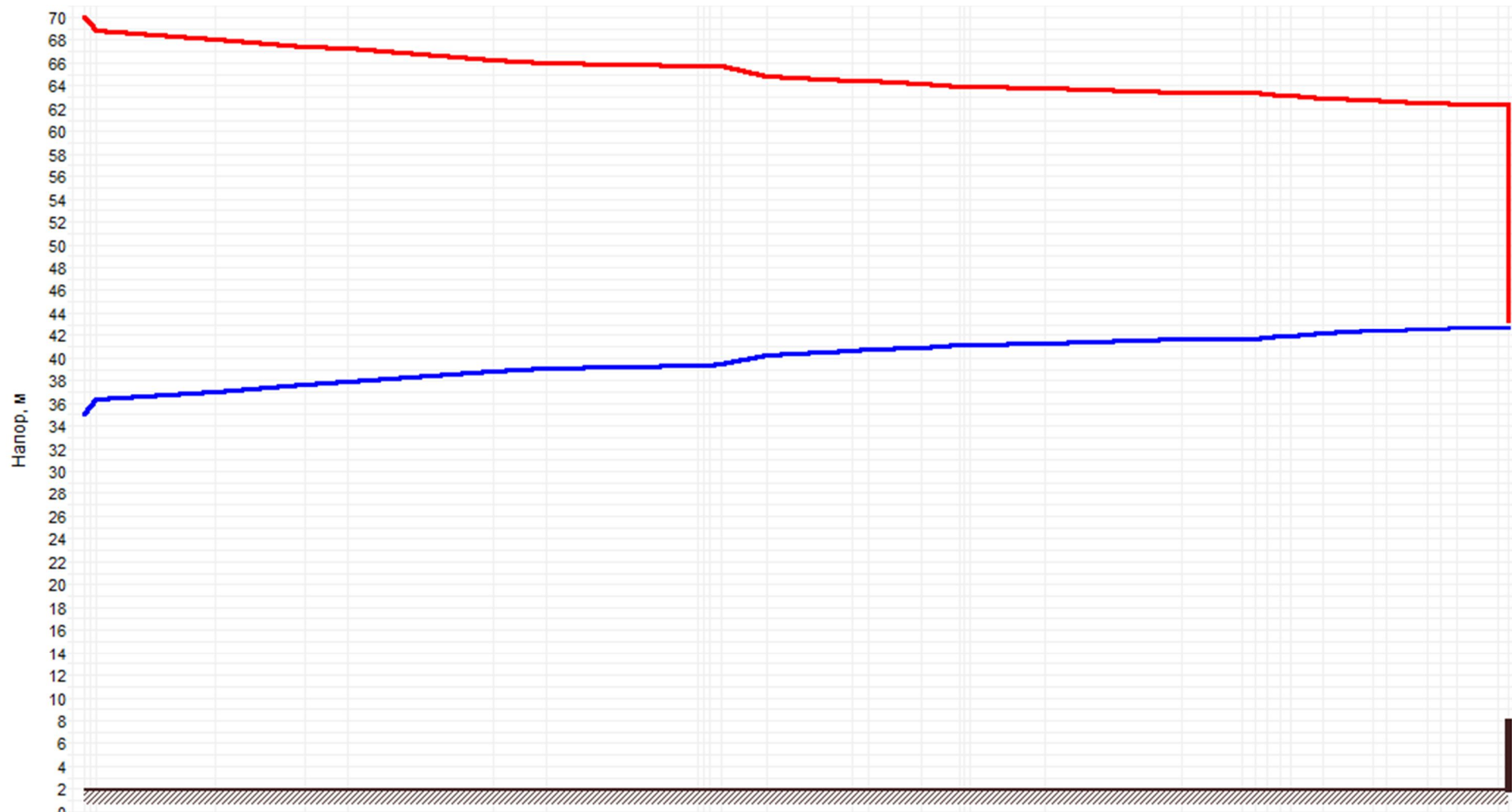
Рисунок 34.4 –График гидравлических режимов рассматриваемого теплопровода
