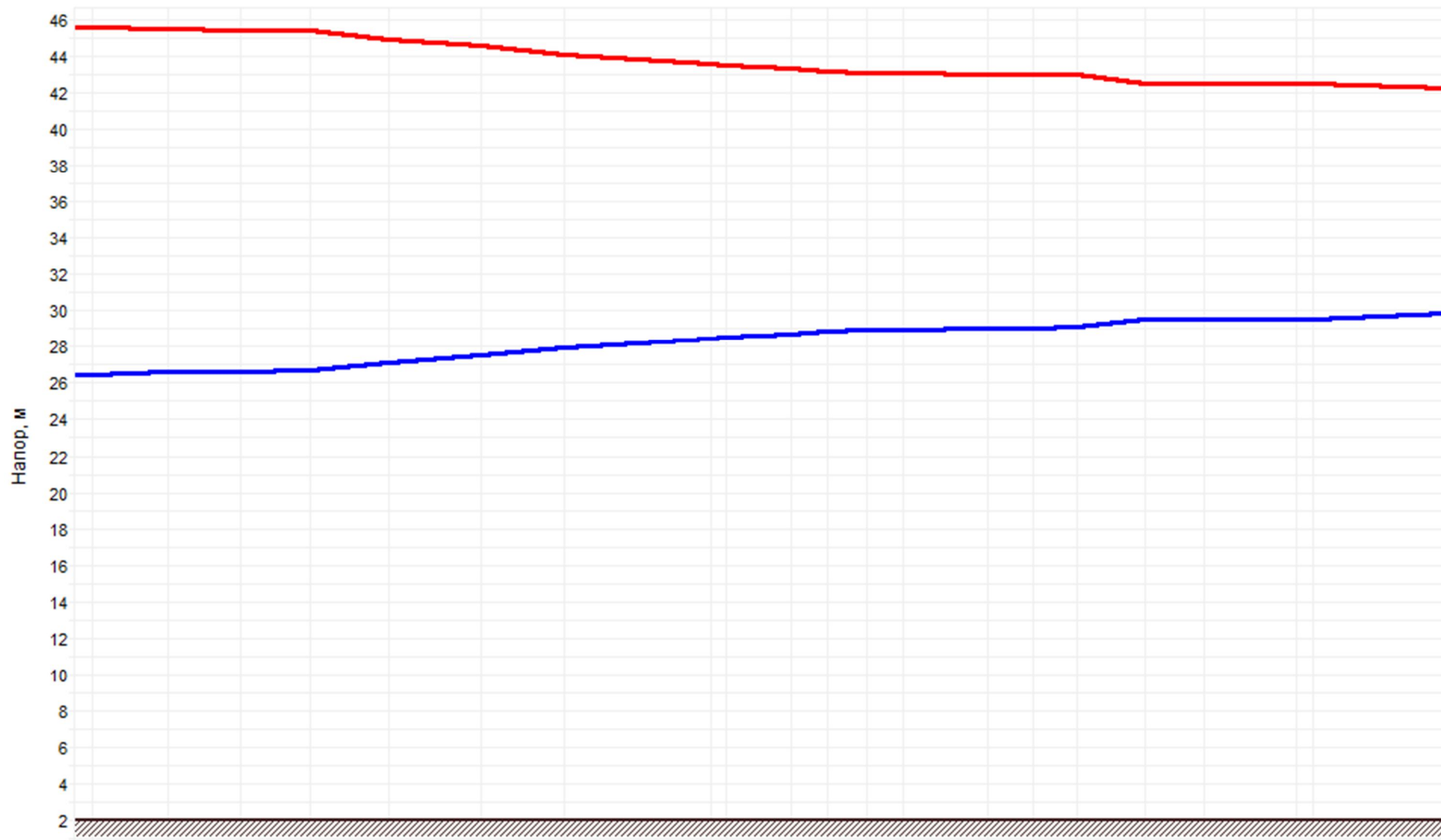
Рисунок 4.2 –График гидравлических режимов рассматриваемого теплопровода
